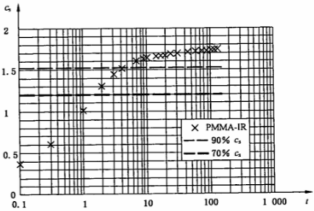
图 B.1 PMMA-IR 的吸水性试验结果
